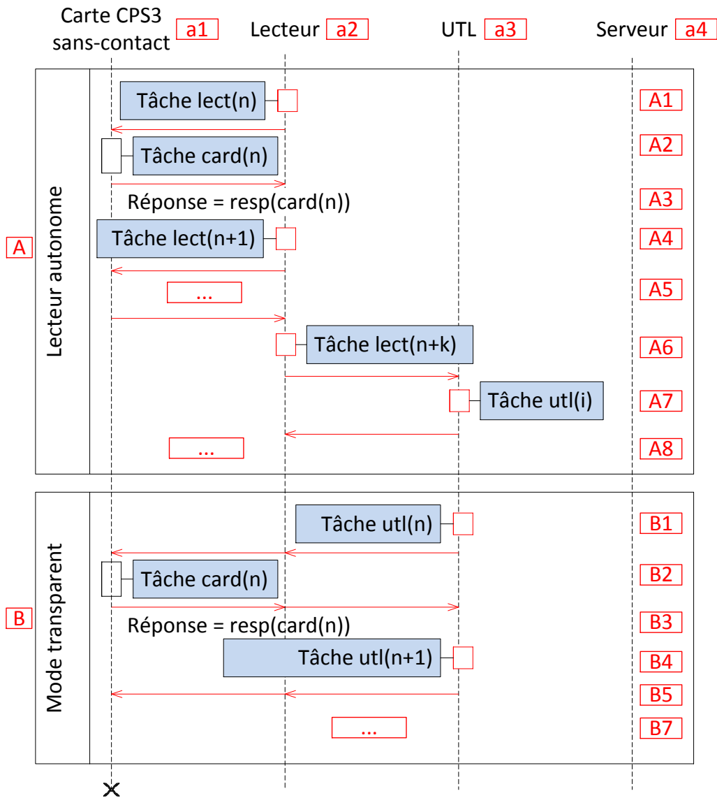
Figure 8 : Différence entre lecteur autonome et lecteur en mode transparent
