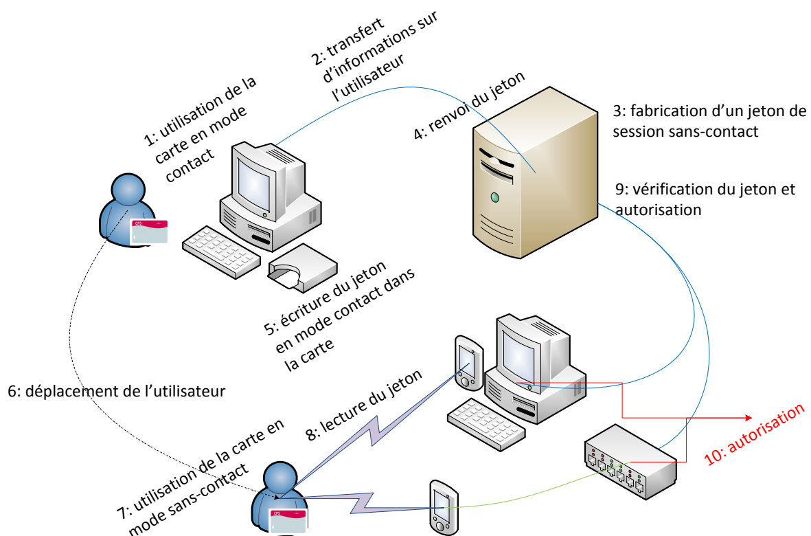
Figure 13 : CPx : Contrôle d'accès avec utilisation de la zone de données carte
