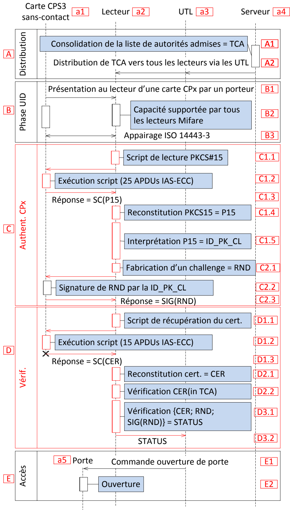
Figure 45 : Diagramme de séquence associé au cas du « lecteur générique IAS-ECC et autonome »
