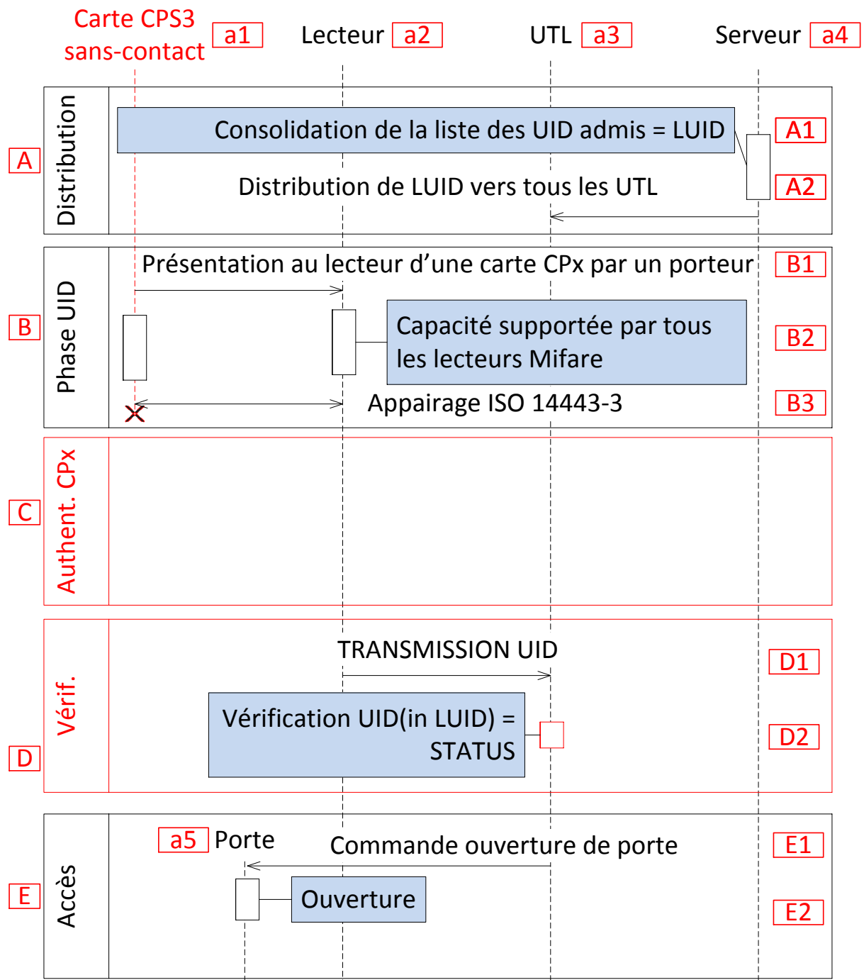
Figure 44 : Diagramme de séquence associé au contrôle d'accès physique en type A sur la base de l'UID Mifare
