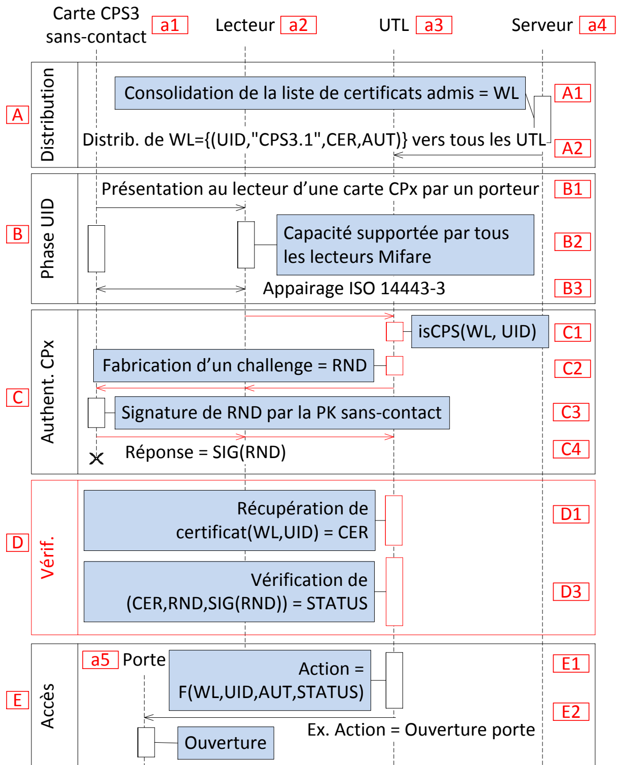
Figure 46 : Diagramme de séquence associé au cas du « lecteur générique IAS-ECC et autonome »
