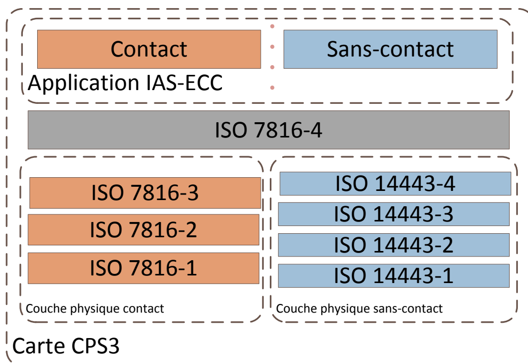
Figure 23 : normes contact / sans-contact rapportées à la CPx
