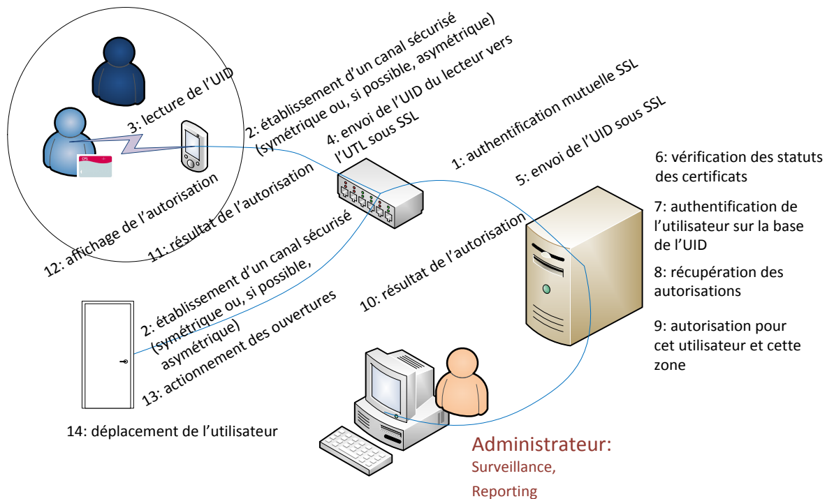
Figure 17 : Exemple d'intégration complète : accès physique : le principe
