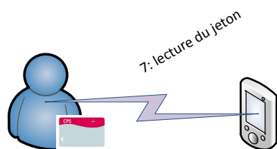
Figure 14 : Remarques Contrôle d'accès avec utilisation de la zone de données carte
