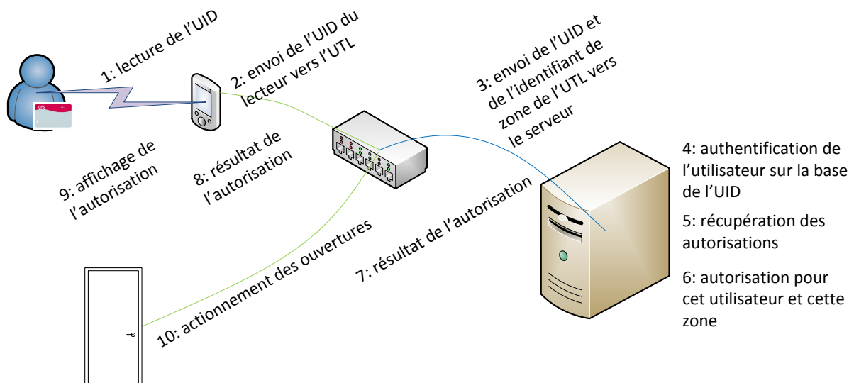
Figure 4 : Principe de l'accès physique type A sur la base de l'UID Mifare
