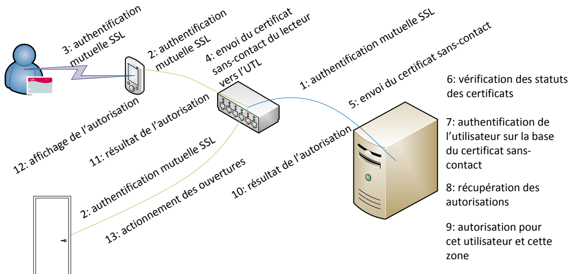
Figure 6 : Principe du contrôle d'accès sans-contact SSL avec la CPS
